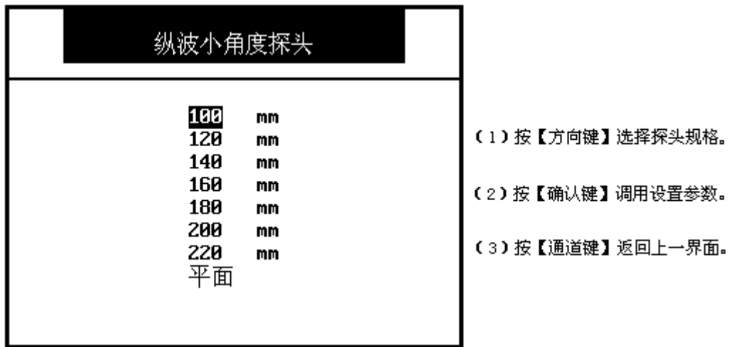
图 11-3 纵波斜探头选择
