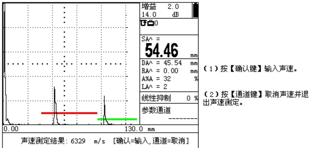
图 11-5 声速测定结果
