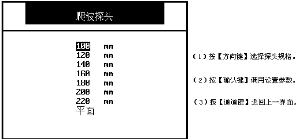
图 11-6 爬波探头选择
