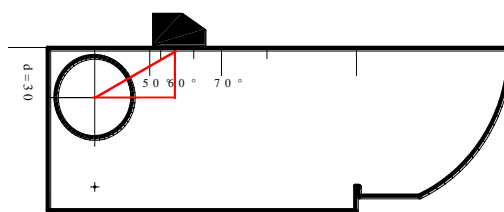
(图 2：校准探头 K 值)
