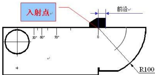
(图 1：校准材料声速、探头零点、探头前沿)
